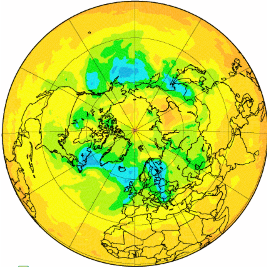
Colonne totale d'ozone (DU) du 01/08/2007
