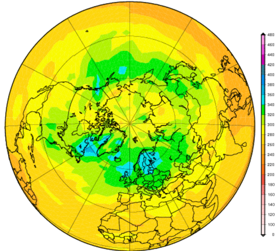
Colonne totale d'ozone (DU) prévue pour le 01/08/2007 à 12 utc
